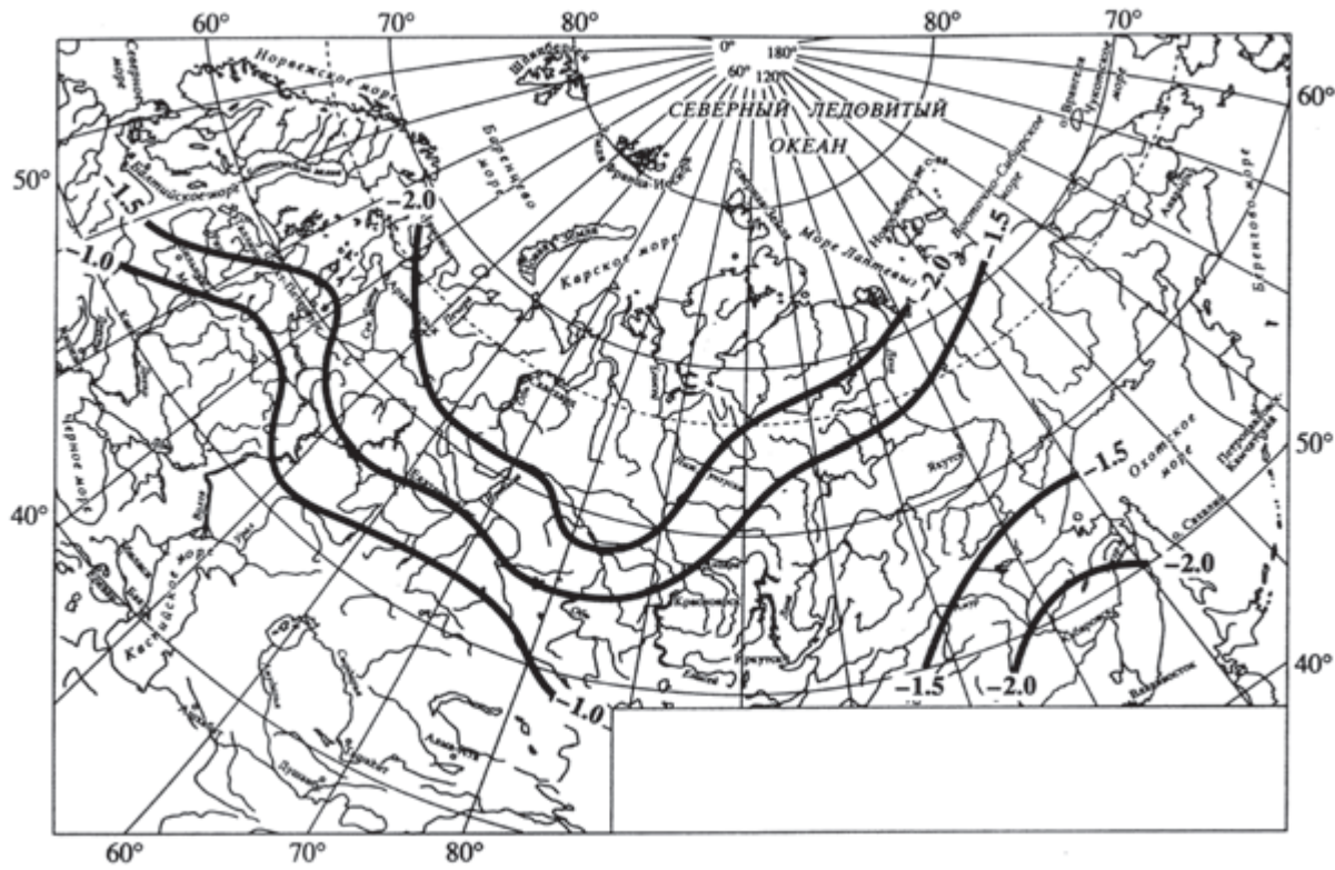
34 Жылдық орташа температураның неогляциаль кезеңі (шамамен 2500 жыл бұрын) мен заманауи мәнін салыстырғандағы ауытқуы ([Климанов, 2002. 3 сур.] бойынша) Deviation of the average temperatures of the year in the neoglacial (about 2500 y.a.) from their current values (on: [Klimanov, 2002. Fig.3]) Отклонение средних температур года в неогляциале (около 2500 л. н.) от современных их значений (по: Климанов, 2002. Рис. 3)
