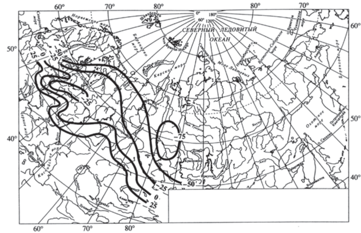
35 Жылдық орташа жауын-шашын көлемінің неогляциаль кезеңі (шамамен 2500 жыл бұрын) мен заманауи мәнін салыстырғандағы ауытқуы ( [Климанов, 2002. 4 сур.] бойынша) Deviation of the average annual amount of precipitation in the neoglacial (about 2500 hp) from their present values (according to: [Klimanov, 2002. Fig.4]) Отклонение средней годовой суммы осадков в неогляциале (около 2500 л. н.) от современных их значений (по: Климанов, 2002. Рис. 4)
